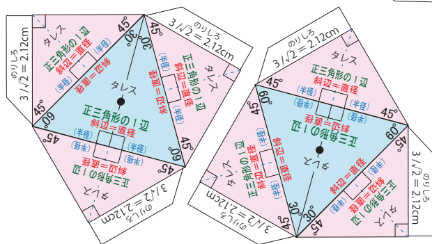
正四角錐（ピラミッド型） 直角正三角錐 × 4 個
